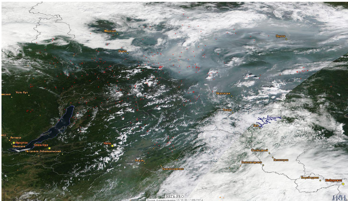
Рис. 1 Пожары в Республике Саха (Якутии), Забайкальском крае, Республике Бурятия
